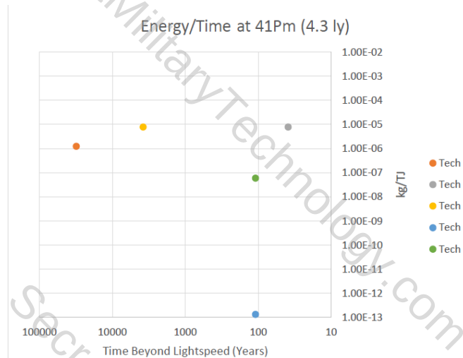
(9c) 270,000 AU (Centauri)
